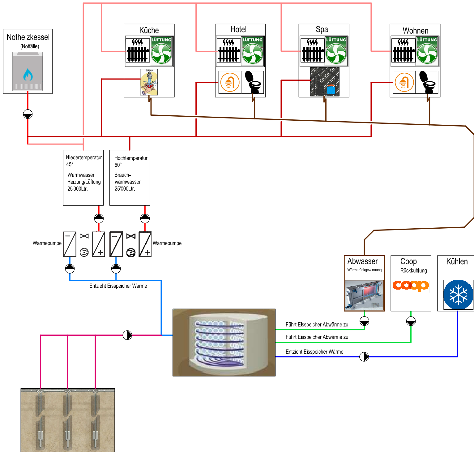
2'340 Meter Erdsonden mit 18 Bohrungen bis in 130m Tiefe.
